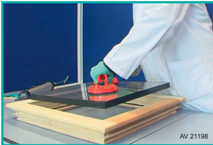
La unidad de vidrio aislante se instala en la hoja de la ventana
