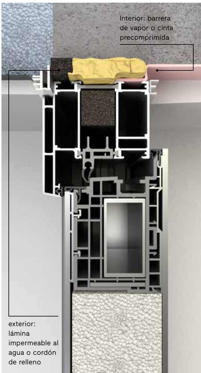
Montaje directo al muro en una fase
